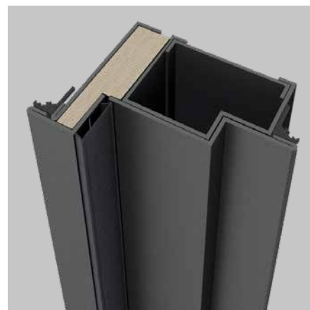
Particolare Telaio a Taglio Termico
